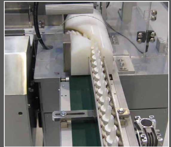
Zuführung für Handeinlage oder automatische Zuführungen
